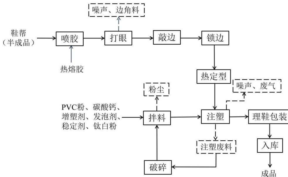
图 2-1 PVC 注塑鞋生产工艺流程及产污环节示意图
