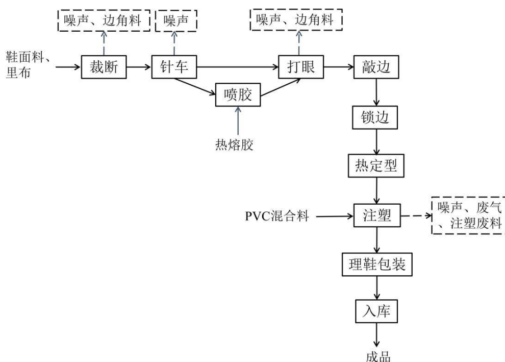
图 2-1 注塑鞋生产工艺流程及产污环节示意图
