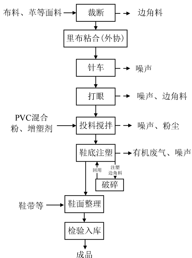
图 2-2 注塑鞋生产工艺
