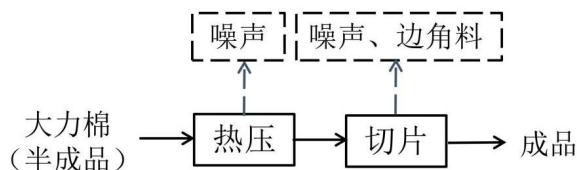
图 2-3 大力棉鞋垫生产工艺流程及产污环节示意图
