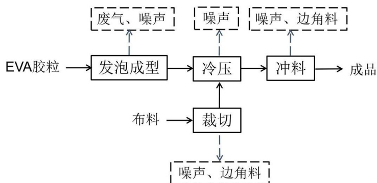
图 2-2 EVA 鞋垫生产工艺流程及产污环节示意图
