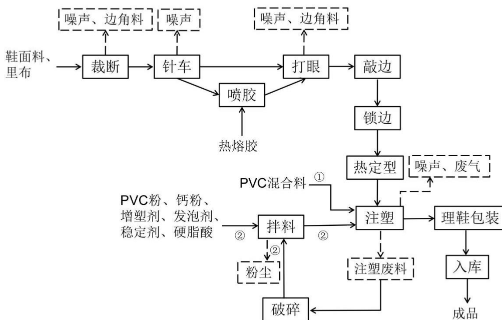
图 2-1 注塑鞋生产工艺流程及产污环节示意图
