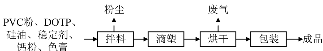
图 2-1 项目生产工艺流程及产污环节示意图
